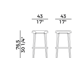
942/AC sgabello \ stool
